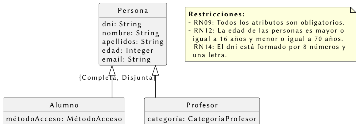
Diagrama de clases - Jerarquía de personas
